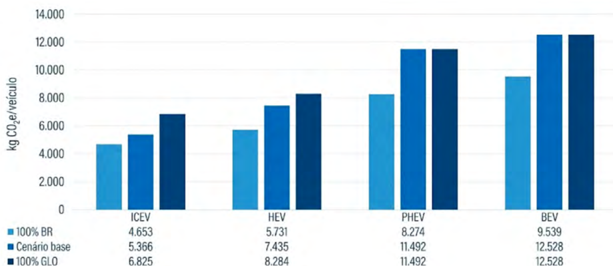
→| Figura 4.12 – Pegada de carbono dos veículos SUV para diferentes cenários de nacionalização
