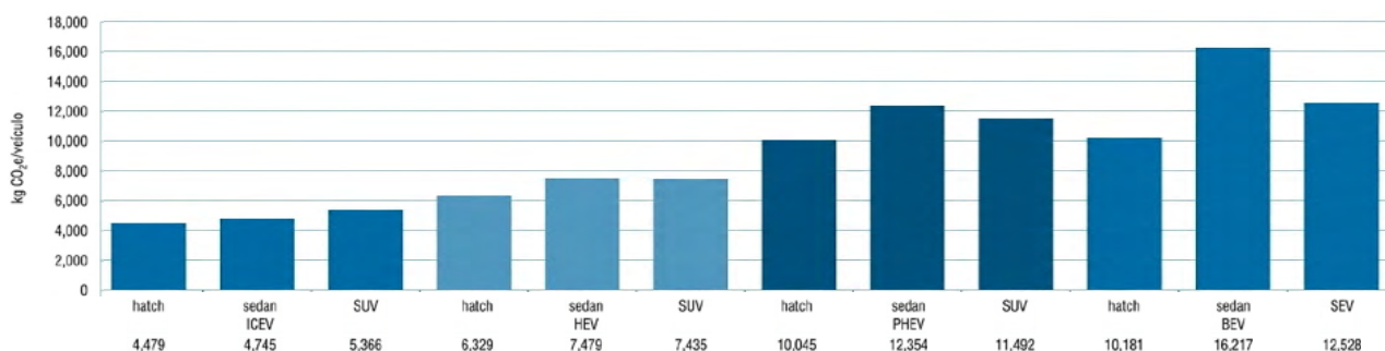
→ Figura 4.7 – Pegada de carbono, do berço-ao-portão, dos doze veículos do Projeto
