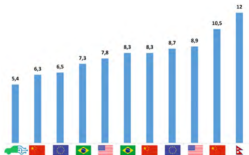
→ Figura 4.15 – Comparação internacional da pegada de carbono do veículo ICEV-SUV em tCO 2 eq/veículo
