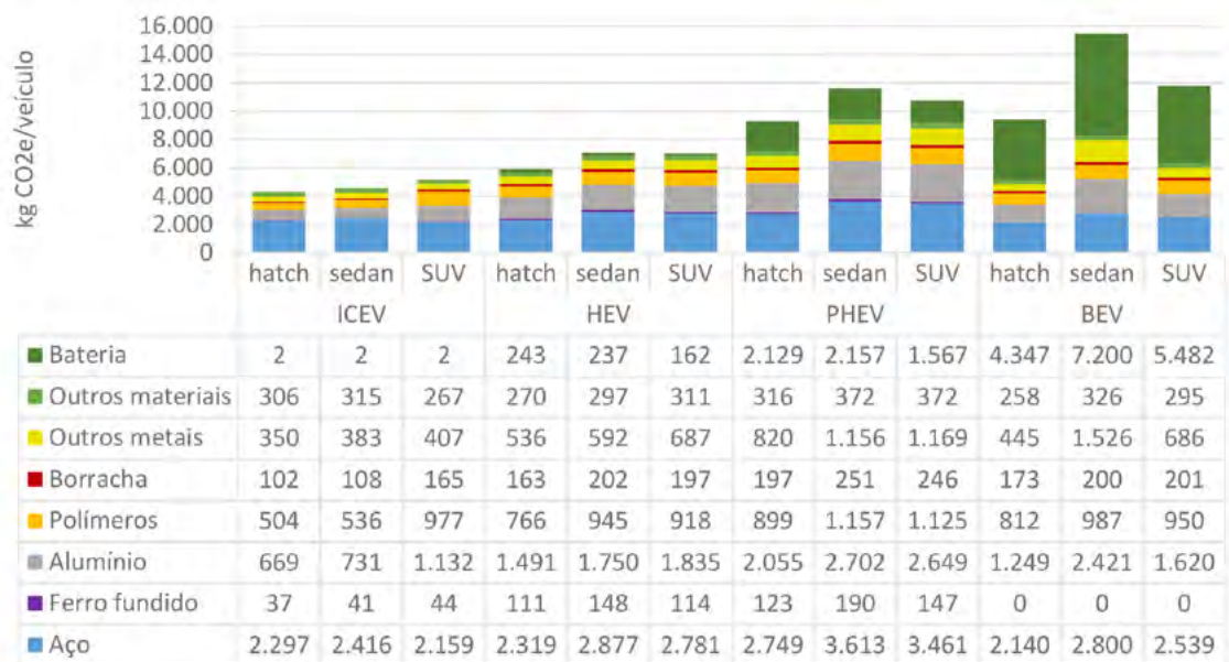
→| Figura 4.9 – Pegada de carbono dos doze veículos avaliados pelo Projeto, por material
