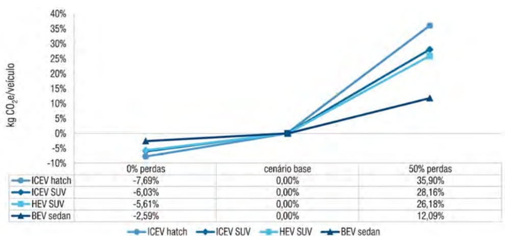
→ Figura 4.14 – Variação da pegada de carbono para o cenário de perdas do aço
