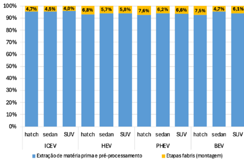
→| Figura 4.8 – Contribuição por etapa do ciclo de vida para a pegada de carbono dos doze veículos do Projeto
