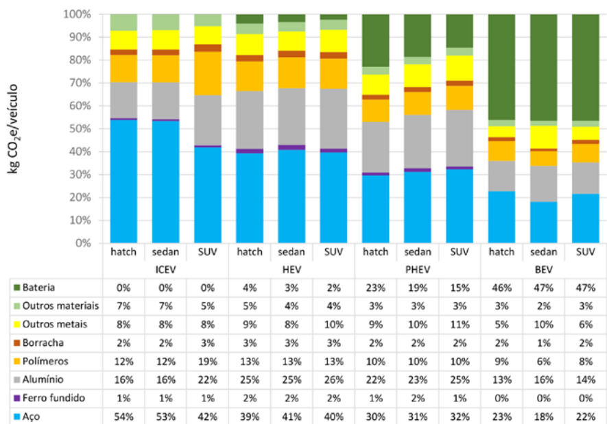
→| Figura 4.10 – Contribuição relativa dos materiais para a pegada de carbono dos doze veículos do projeto
