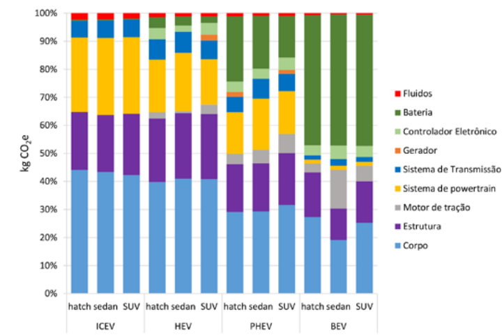
→ Figura 4.11 – Contribuição dos sistemas dos veículos para a pegada de carbono, do berço- ao- portão
